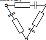
Dreieckschaltung
